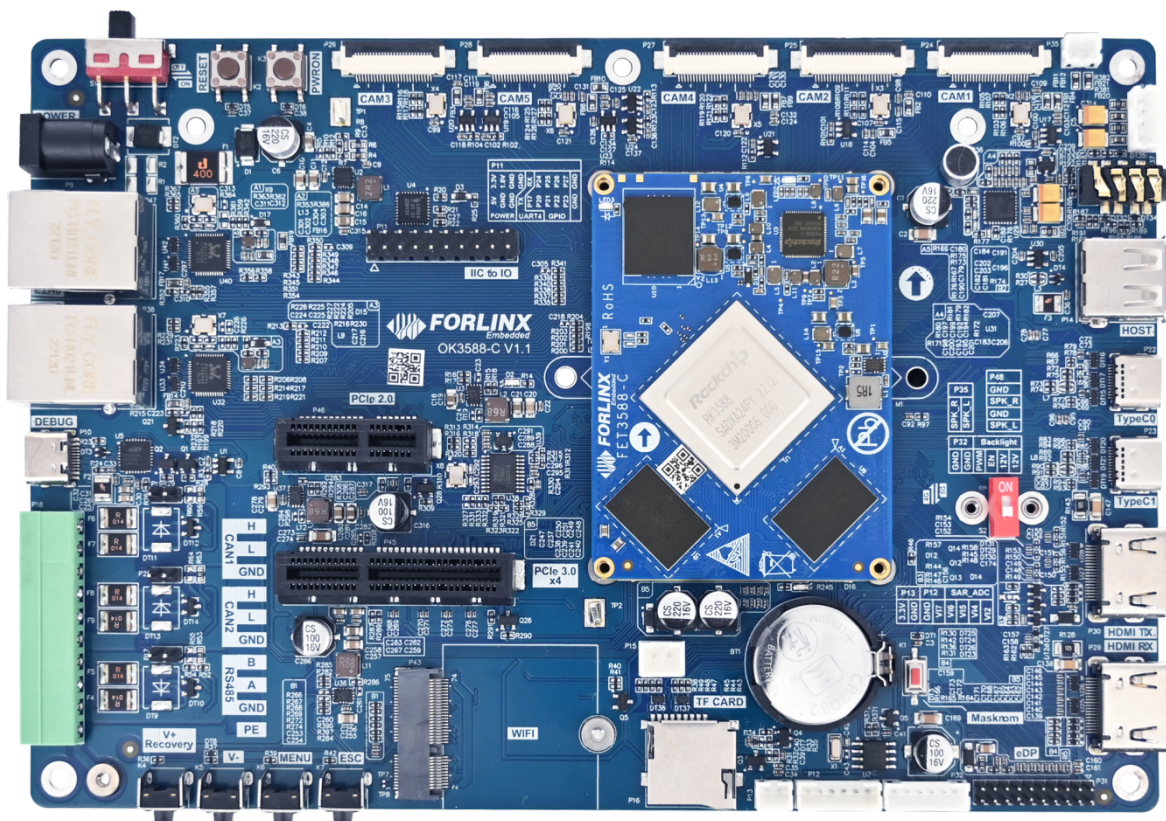
OK3588-C 开发板
