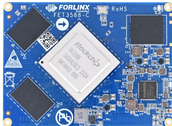
FET3588-C 核心板
